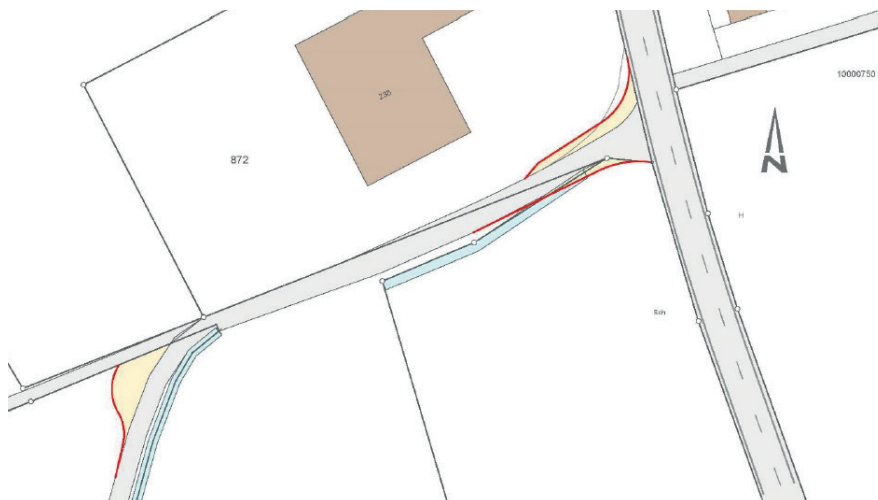
Abb. 8 Planausschnitt Machbarkeitsstudie «Erschliessung Camping Steibüel»; Quelle: Viaplan AG, Sursee
