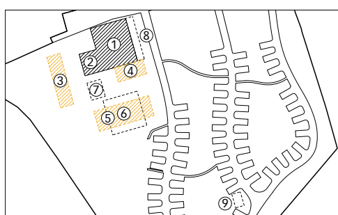
Abb. 4 Konzeptplan «Gebäude»
